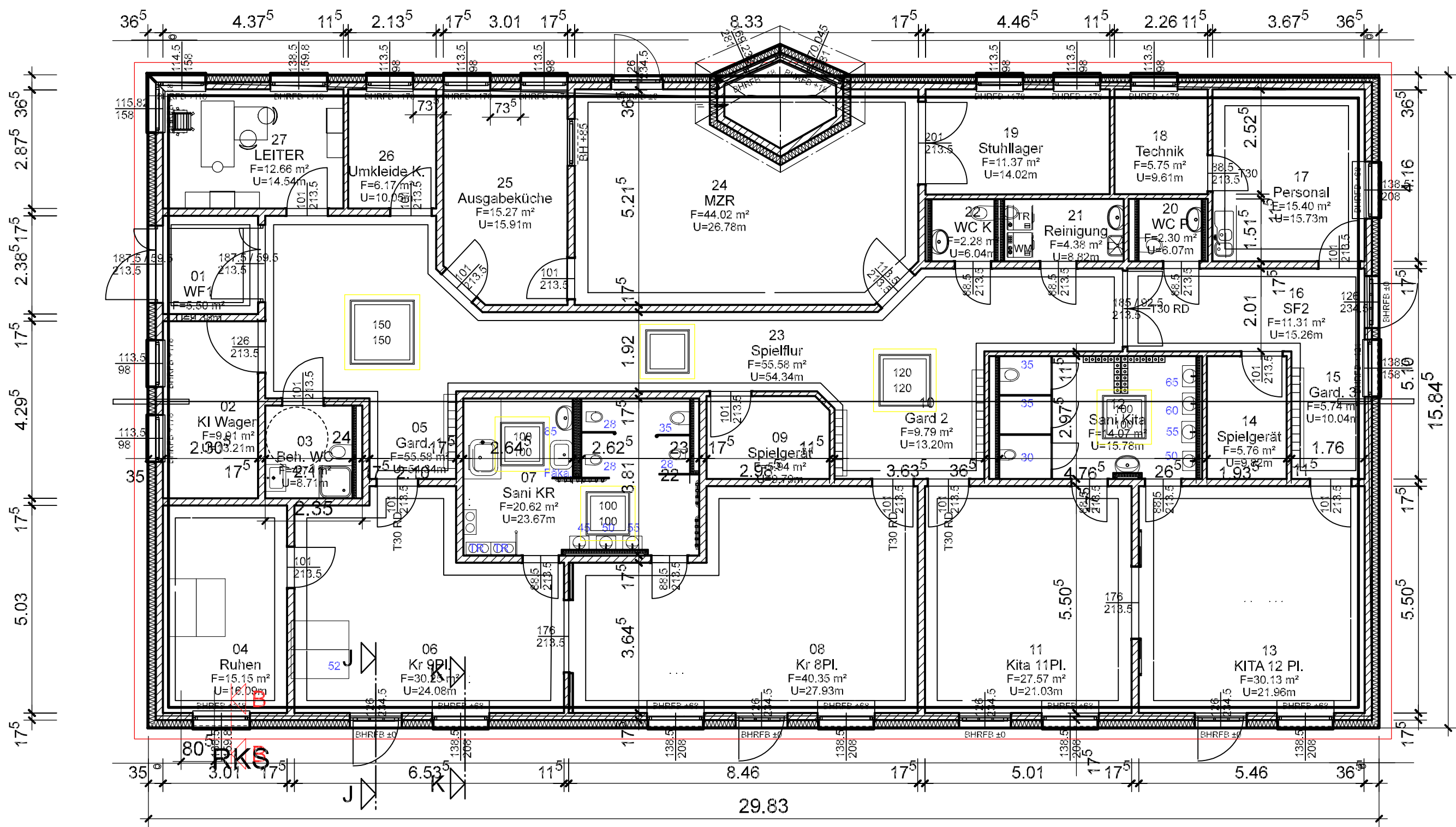
Grundriss M1:100 - Raumprogramm- Neubau KITA 40 Plätze Lindenallee in Hansestadt Stendal OT Uenglingen
