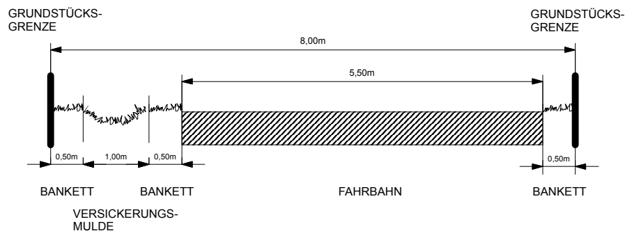
Bild 1: Strassenquerschnitt
