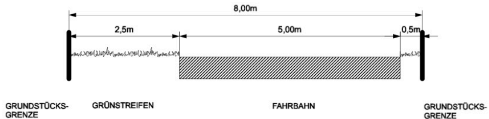
Bild 1: Strassenquerschnitt
