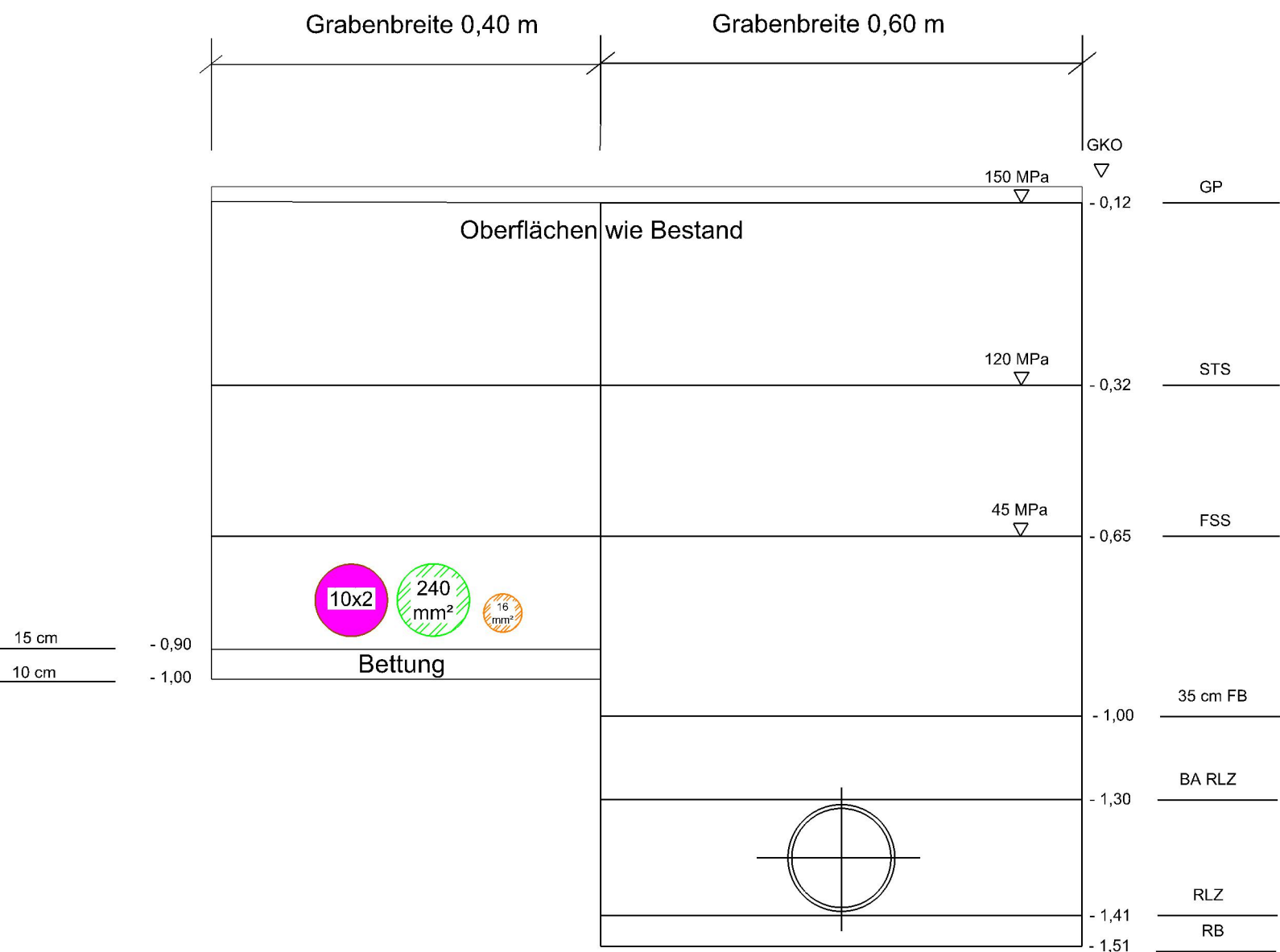
Grabenprofilschnitt
